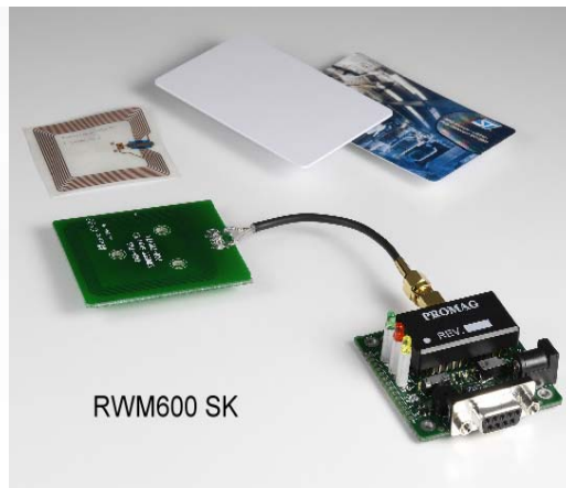
RWM600 Reader Module
